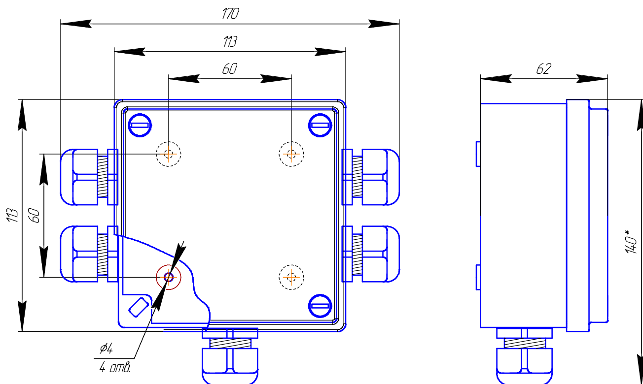
Масса не более 0,26 кг Степень защиты IP56 Тип и количество сальников оговаривается при заказе Сумматор сигнала СС-24-К2, СС-24-К4
