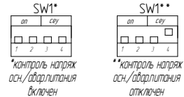
Варианты выставление DIP перкл. на силовом блоке БС КФ-6:
