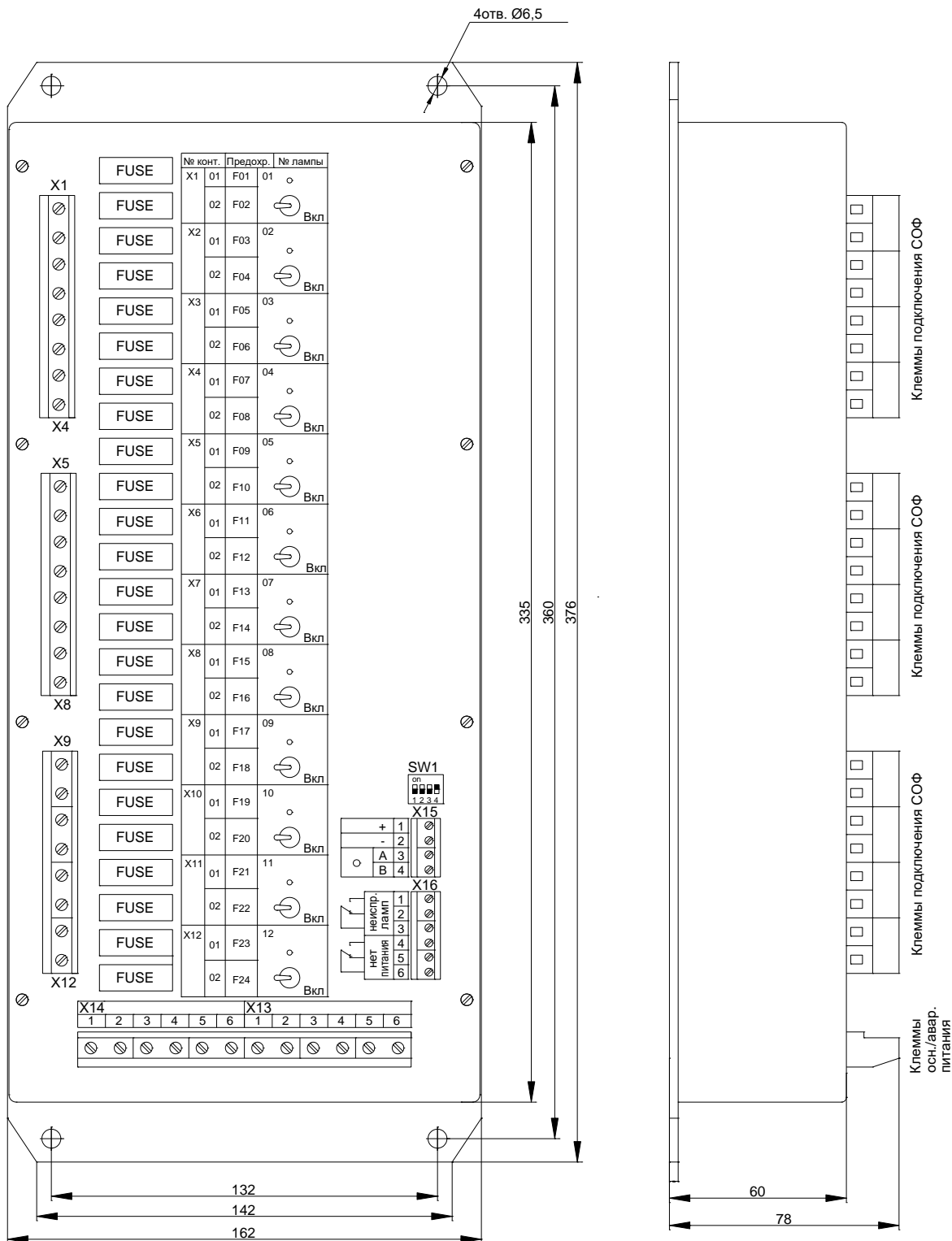
Блок силовой БС КФ-220-12
